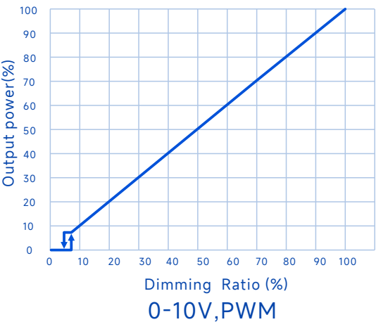
输出功率Vs.调光信号
